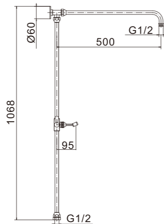
PS2011 Rigid riser kit
